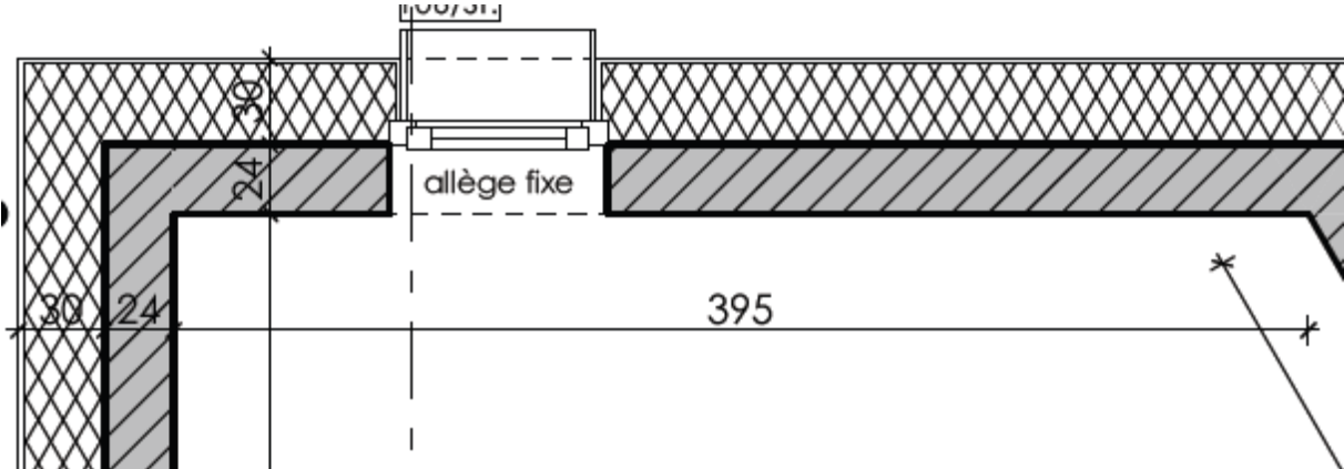
Mur 2 : 395 x 250
